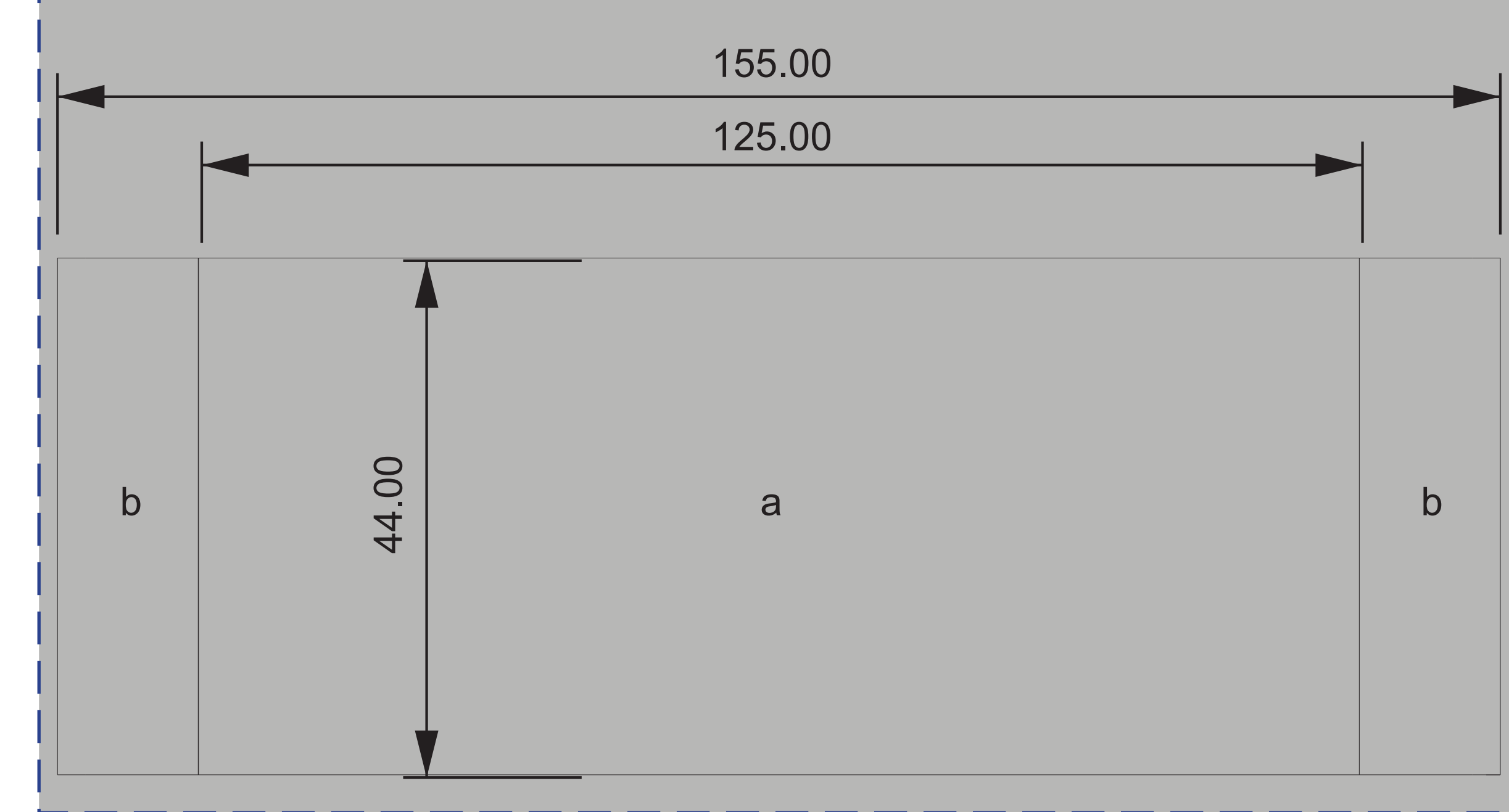
RZUT SKALA 1:5
